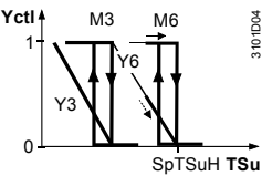
Функциональная диаграмма
