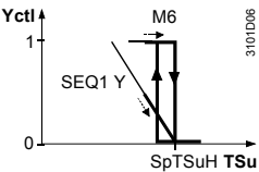
Функциональная диаграмма
