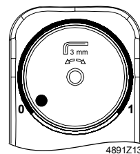
Индикатор положения, позиция 0: Клапан закрыт
